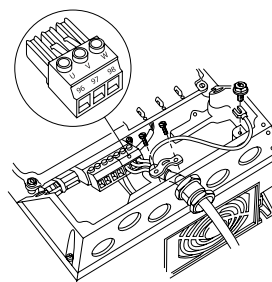
Рисунок 3.10: Подключение двигателей, типоразмер A4/A5 (IP 55/66/NEMA тип 12)
