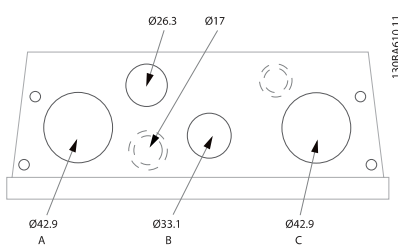
Рисунок 3.17: Отверстия ввода кабелей для типоразмера B2. Предлагаемое использование отверстий является рекомендуемым, но не единственно возможным решением.
