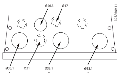
Рисунок 3.16: Отверстия ввода кабелей для типоразмера B1. Предлагаемое использование отверстий является рекомендуемым, но не единственно возможным решением.
