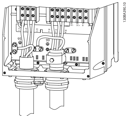
Рисунок 3.14: Подключение двигателей, типоразмер C1 и C2 (IP 21/ NEMA тип 1 и IP 55/66/ NEMA тип 12)
