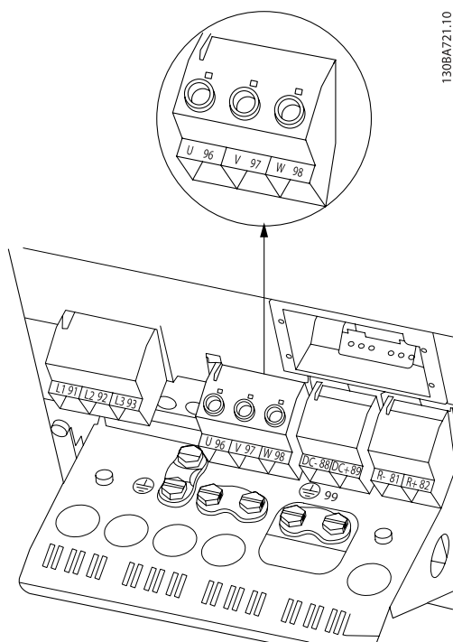
Рисунок 3.13: Подключение двигателей, типоразмер B4 .
