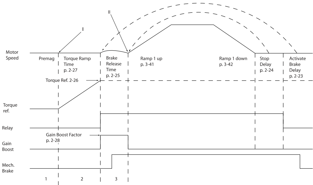
Рисунок 4.1: Последовательность отпущания тормоза при управлении механическим тормозом подъемного механизма I) Задержка включения тормоза: Преобразователь частоты начинает снова с положения задействованного механического тормоза . II) Задержка останова: Когда время между последовательными запусками короче, чем настройка в пар. 2-24 Stop Delay , преобразователь частоты запускается без применения механического тормоза (например, реверс).
