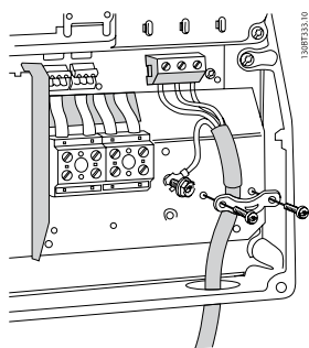
Рисунок 3.11: Подключение двигателей, типоразмер B1 и B2 (IP 21/ NEMA тип 1, IP 55/ NEMA тип 12 и IP66/ NEMA тип 4X)
