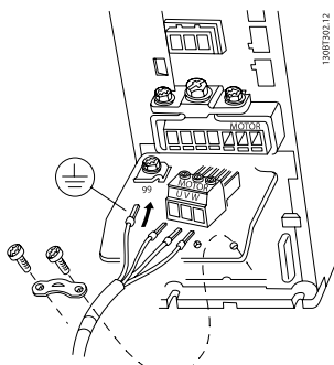
Рисунок 3.9: Подключение двигателей, A1, A2 и A3
