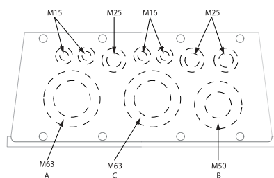
Рисунок 3.18: Отверстия ввода кабелей для типоразмера C1. Предлагаемое использование отверстий является рекомендуемым, но не единственно возможным решением.
