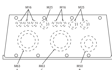
Рисунок 3.19: Отверстия ввода кабелей для типоразмера C2. Предлагаемое использование отверстий является рекомендуемым, но не единственно возможным решением.
